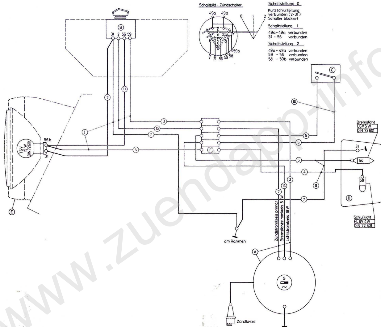
Schaltbild - Zündschalter
