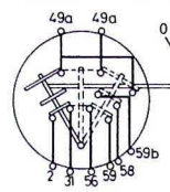
Schaltbild - Zündschalter
