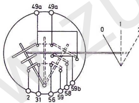
Schaltbild - Zünd - Lichtschalter
