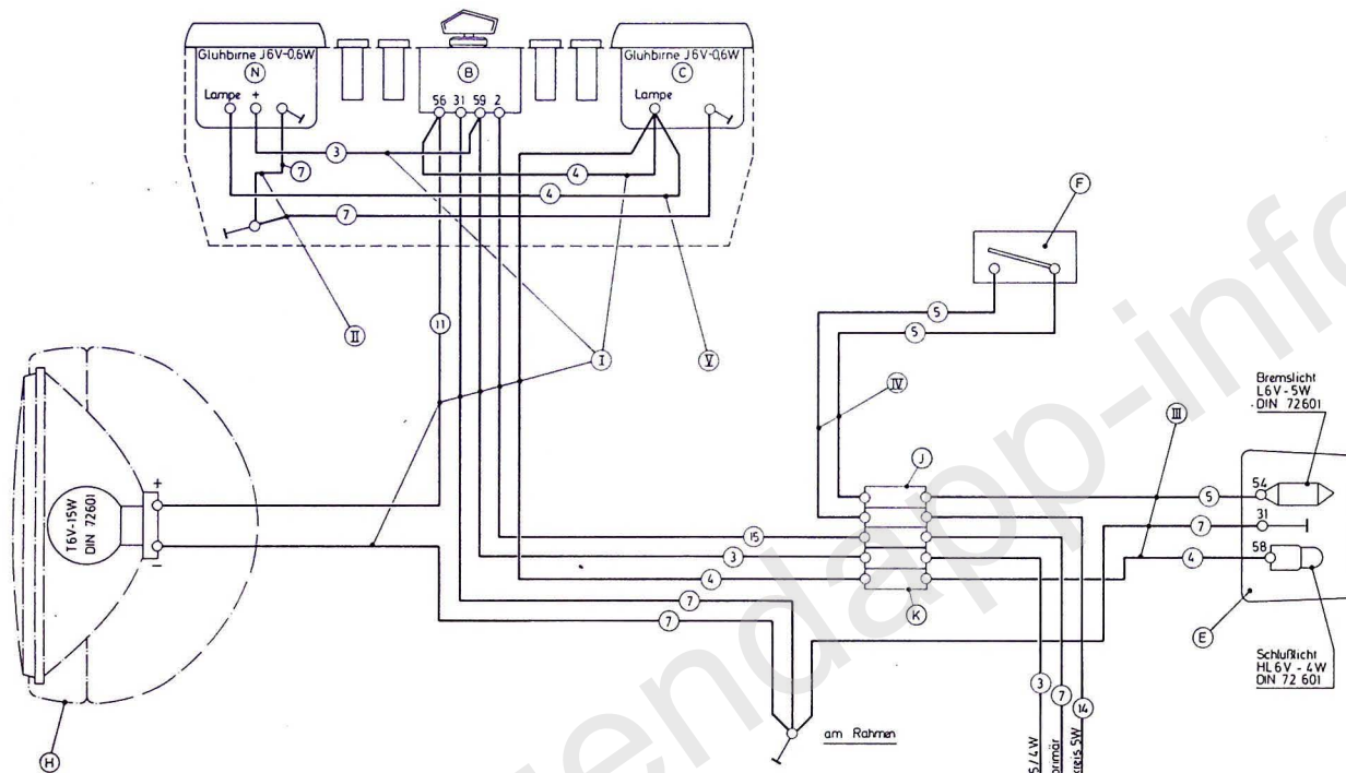
Schaltbild - Zünd - Lichtschalter
